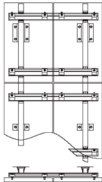
DWG 3 – Outer Edge
