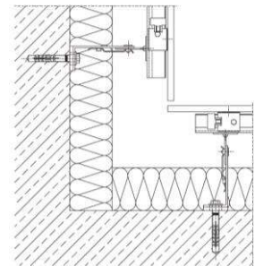
DWG 2 – Inner Edge
