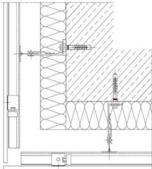
DWG 3 – Outer Edge
